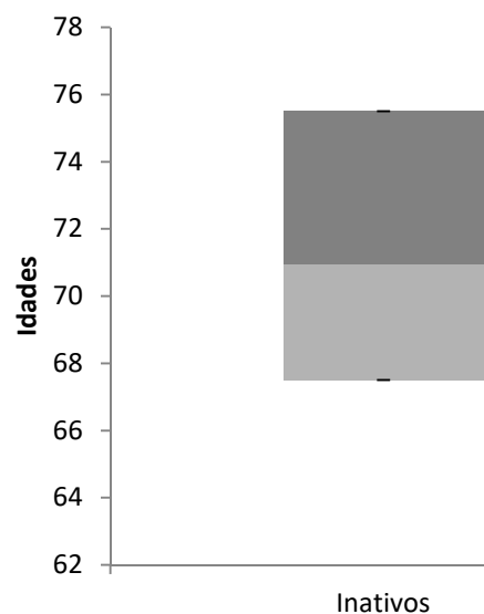
BOXPLOT INATIVOS
